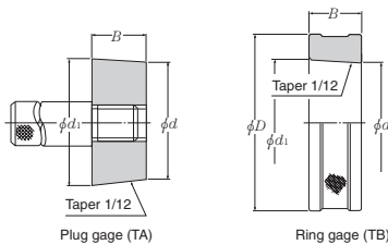
Fig. 6.29 Taper gage
