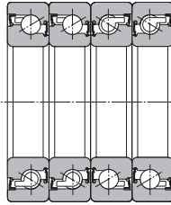
When two rows bear axial load (DTBT)
